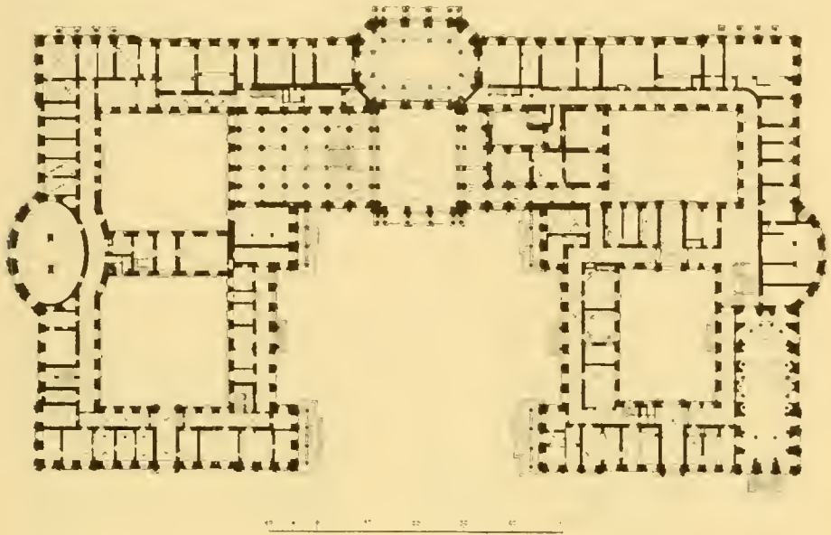
Fig. 107. Residenz zu Würzburg. Grundriss des Erdgeschosses.
